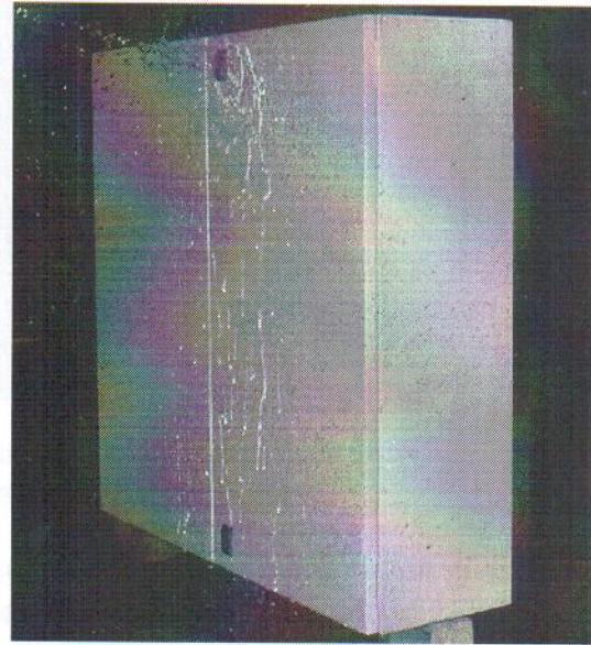
Сварной навесной двухдверной шкаф серии CE(800x1000x300) мм
